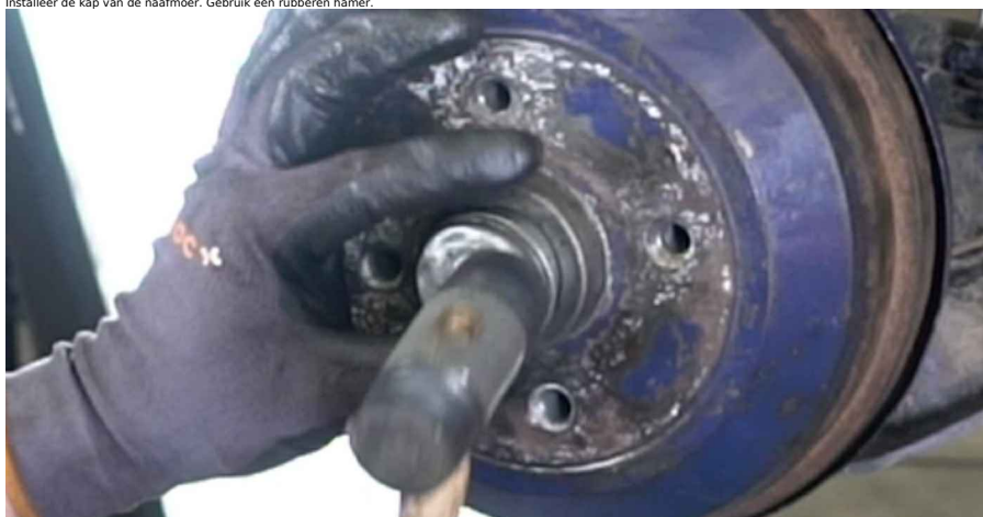
35 Behandel het contactvlak waar de velg met de remtrommel in aanraking komt met een daarvoor bedoeld middel. Maak gebruik van keramisch vet.
