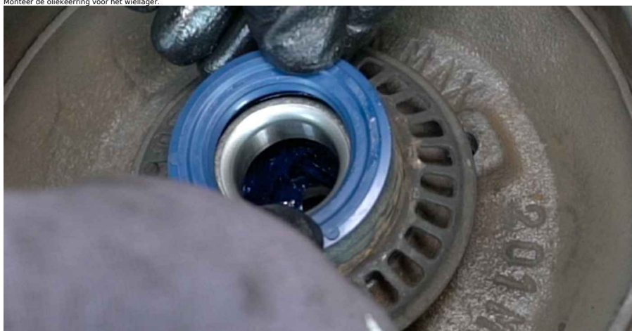
23 Behandel de asstomp. Gebruik allesreiniger. Gebruik lagervet.
