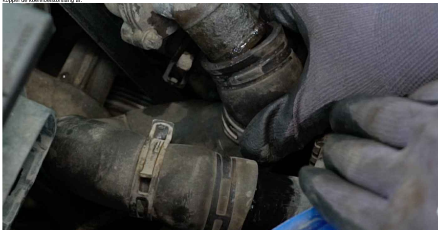
Vervanging: thermostaat - VAUXHALL Combo Mk I (B) Van (593). AUTODOC beveelt aan:
