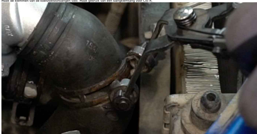
30 Reinig de verbindingen van de koelvloeistofslang. Gebruik allesreiniger.
