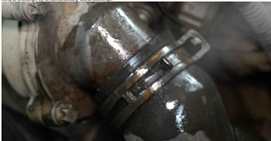
16 Maak de klemmen van de koelvloeistofslangen los. Maak gebruik van een slangklemtang voor Clic-R.
