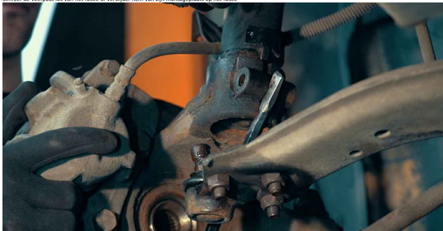
Vervanging van de stofhoes en het aanslagrubber op een veerpoot
