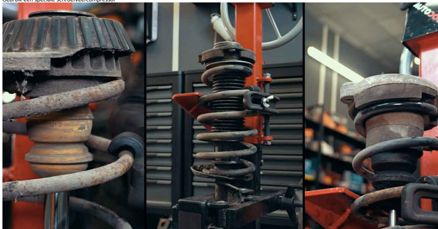
13 Verwijder de bovenste veerpotsteun om bij de stofhoes en het aanslagrubber te komen
