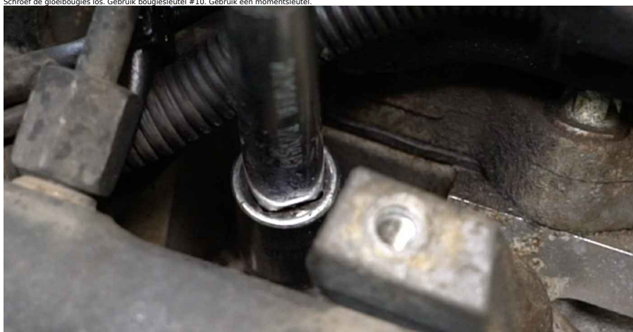
12 Schroef de gloibougies los. Gebruik bougiesleutel #10. Gebruik een momentsleutel.
